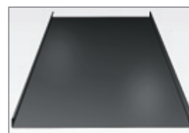
Stavební šíře 535 nebo 595 mm dle šířky suroviny
