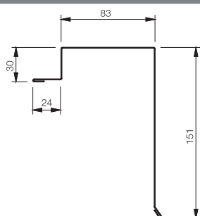
VISRP25 Závětrná lišta – vrchní, dl. 2000 mm
