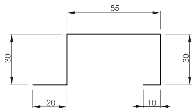
C1SRP25 Hřebenový/nároční profil nevětráný, dl. 2000 mm
