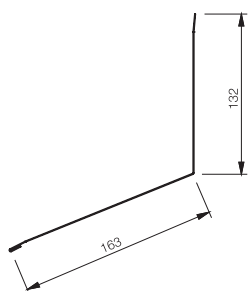
VISRP25 Závětrná lišta – vrchní, dl. 2000 mm
